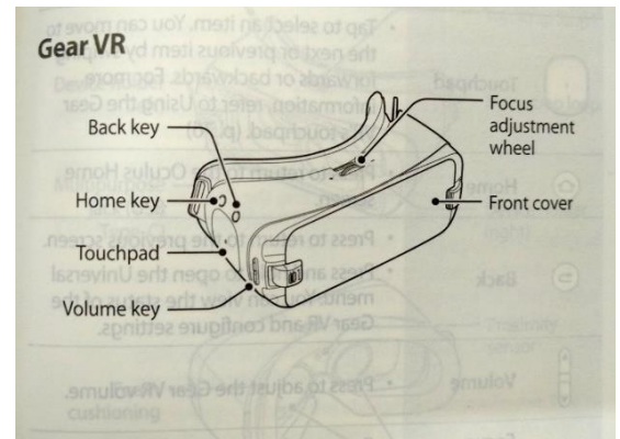
Figura 41- Componentes de las gafas RV
